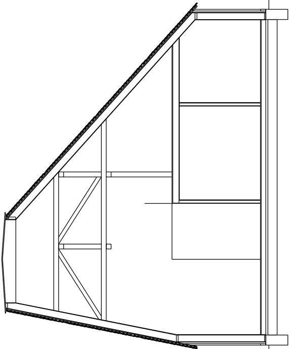
N-S Schnitt
