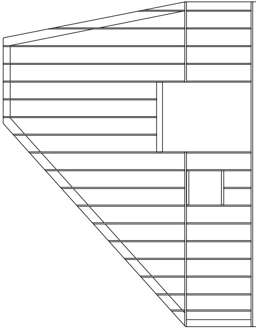
Straßenseite, Holzrahmenkonstruktion
