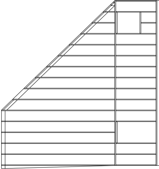
Hofseite, Holzrahmenkonstruktion
