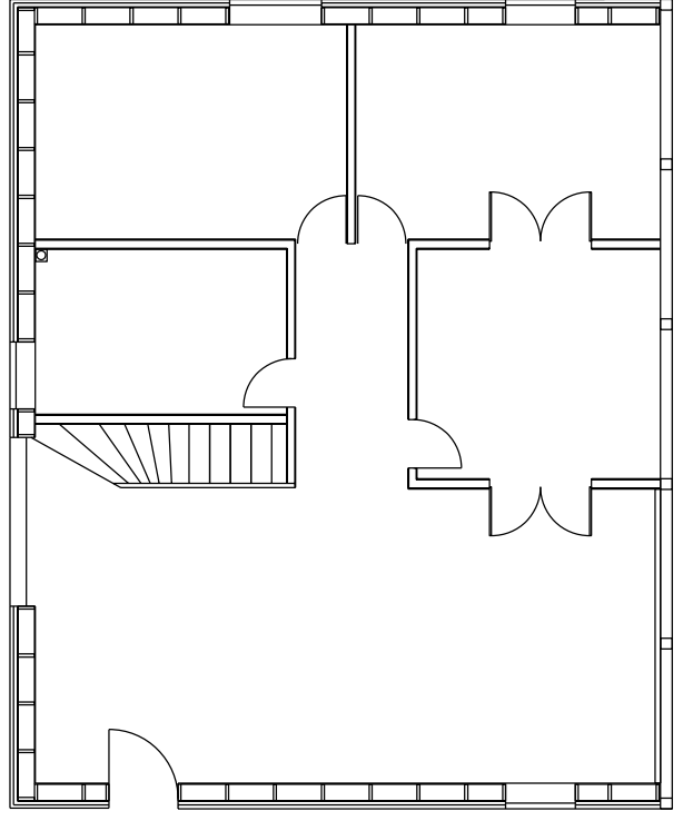
Erdgeschoss, Holzrahmenkonstruktion
